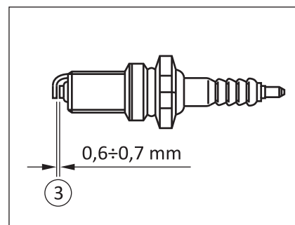
3. Przerwa na świecy zapłonowej 0,6÷0,7 mm. Ustaw przerwę wg tej normy
