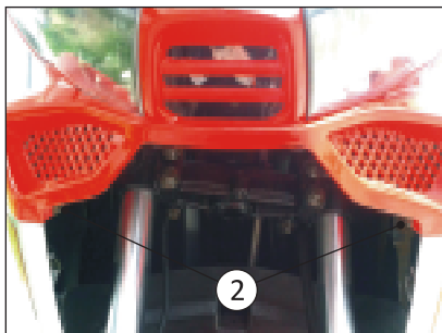
Odkręć wkręty (2)
