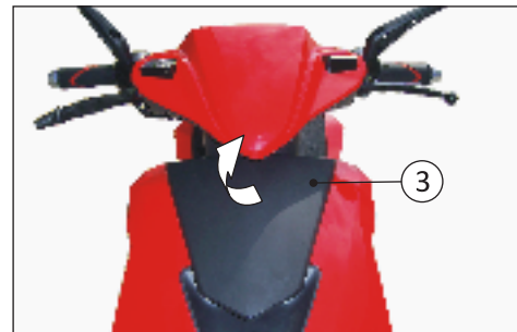
Zdejmij pokrywę (3)
