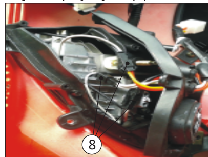
Rozepnij złączki (8)
