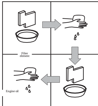
Wkład filtra
