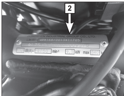
2. Tabliczka znamionowa jest przynitowana na główce ramy po lewej stronie
